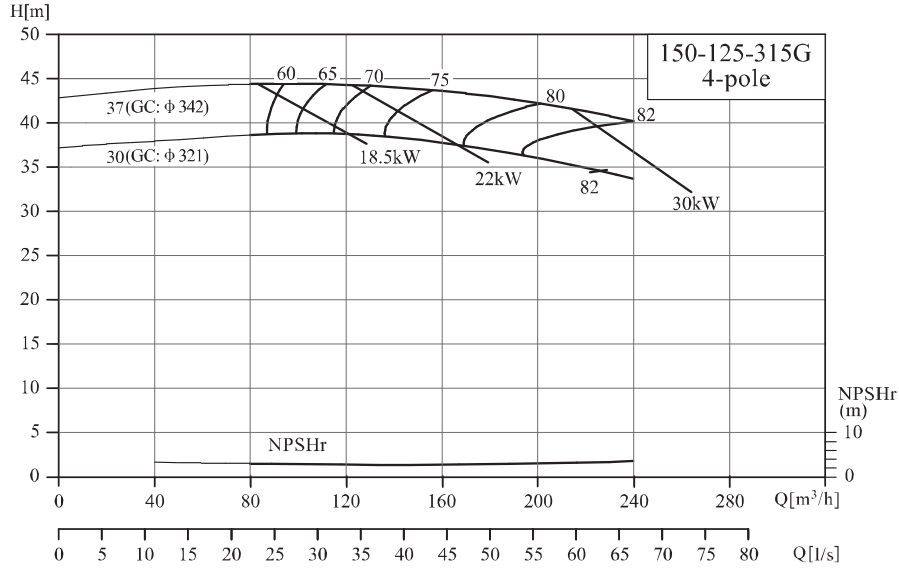
NIS/NISF150-125-315G/150-125-400(Q)
