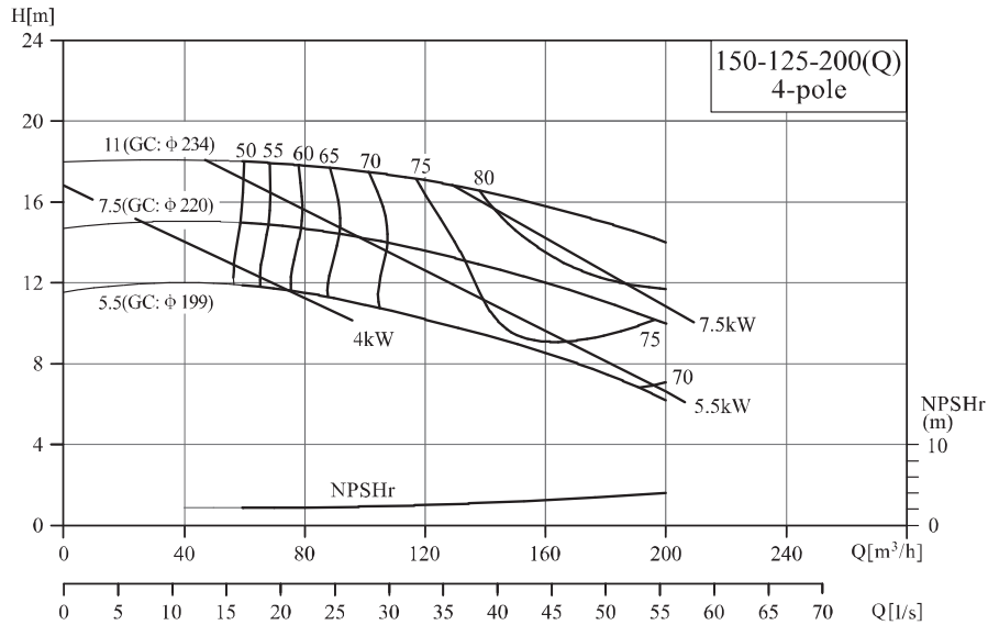
NIS/NISF150-125-200(Q)/150-125-200G
