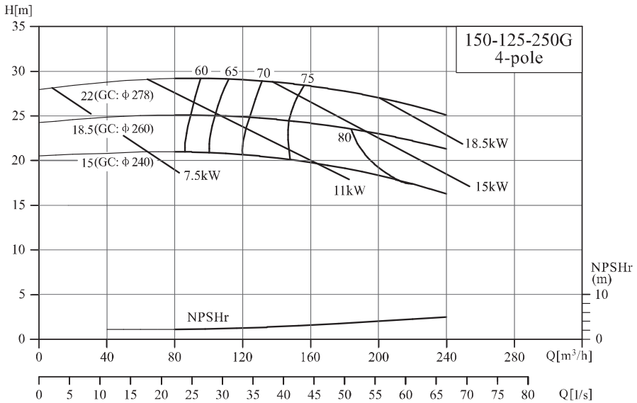
NIS/NISF150-125-250G/150-125-315(Q)
